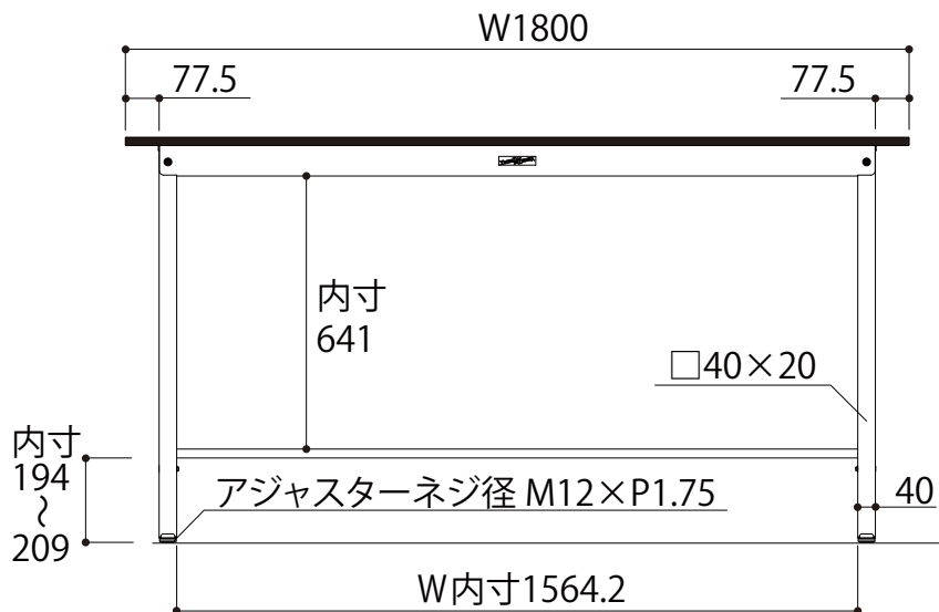
正面図
