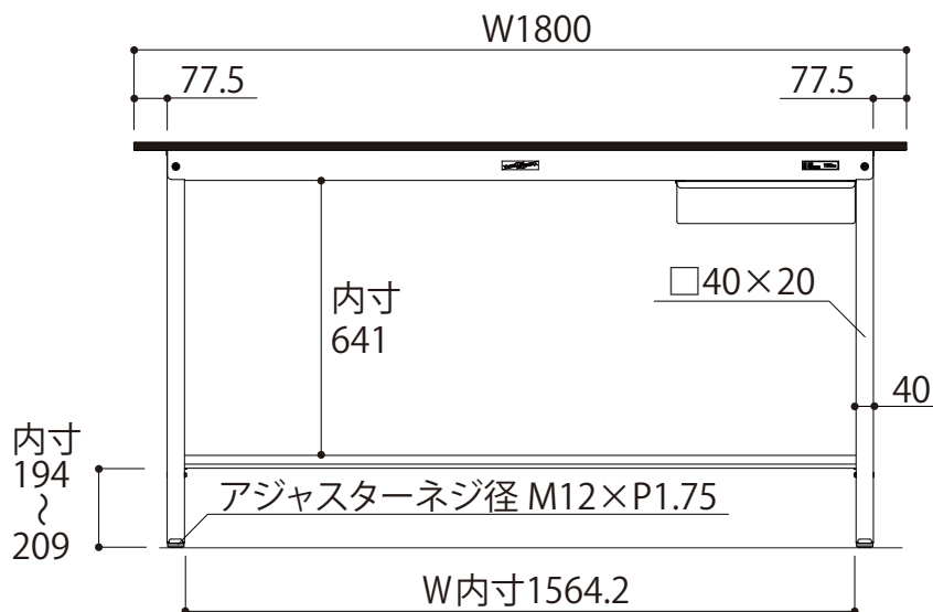
正面図
