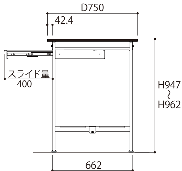
側面図
