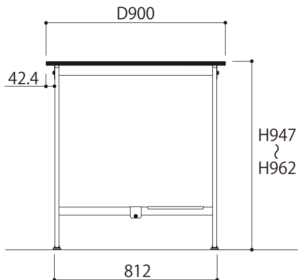
側面図
