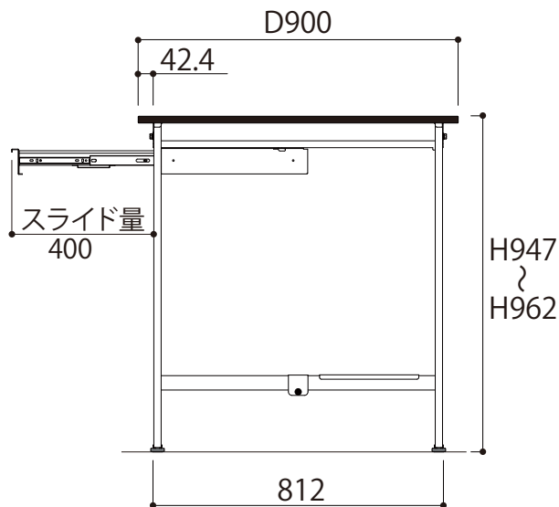
側面図
