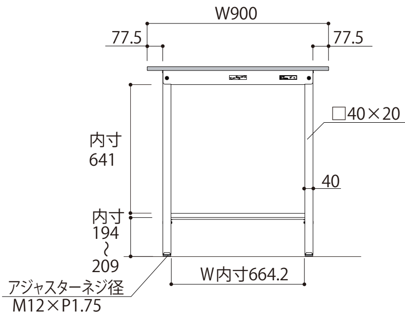
正面図
