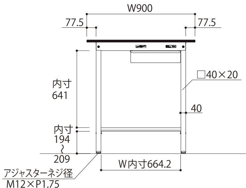
正面図
