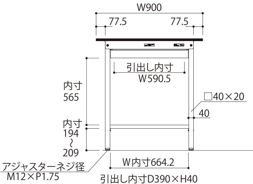
正面図
