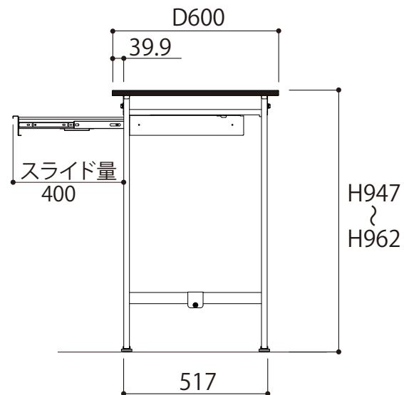
側面図
