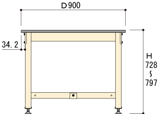
側面図
