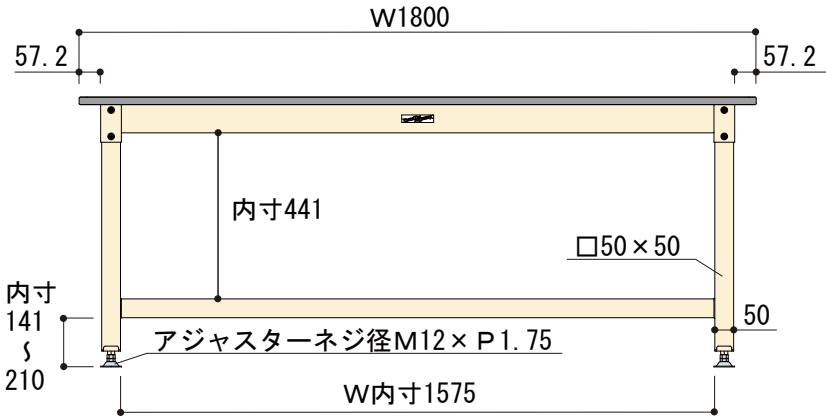
正面図
