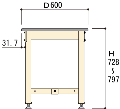
側面図
