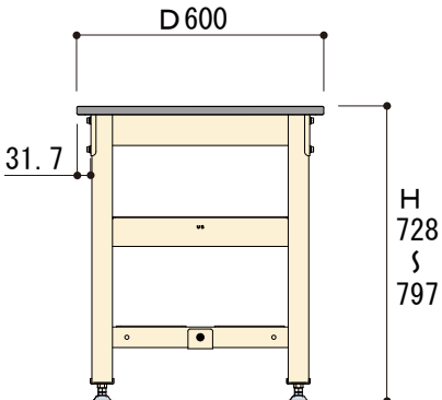
側面図
