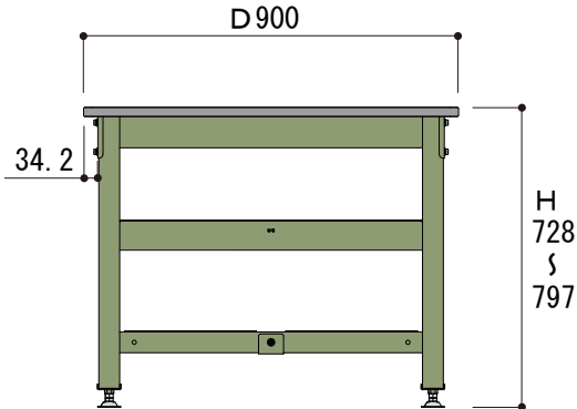
側面図
