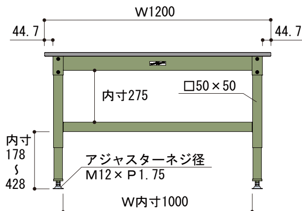
正面図
