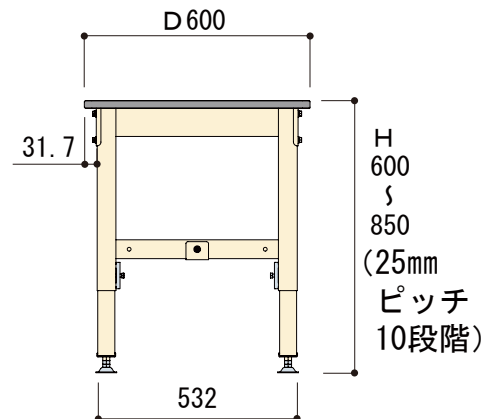
側面図
