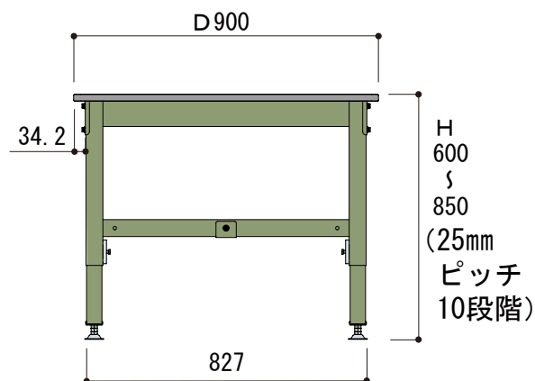
側面図
