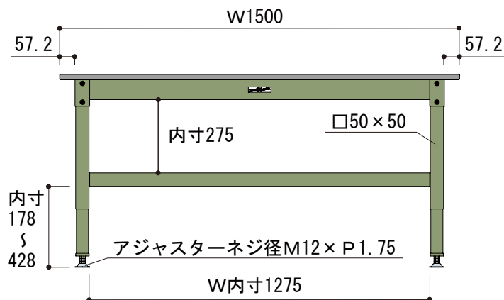
正面図
