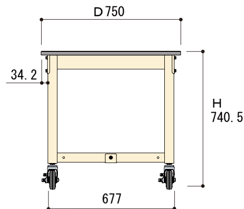
側面図
