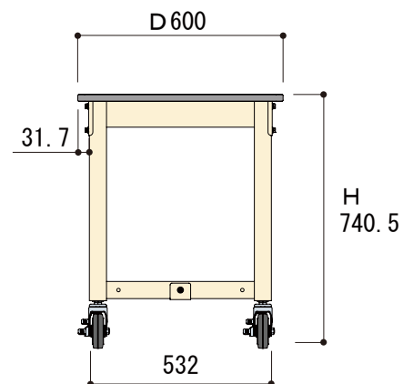
側面図
