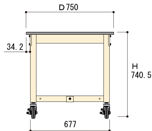
側面図
