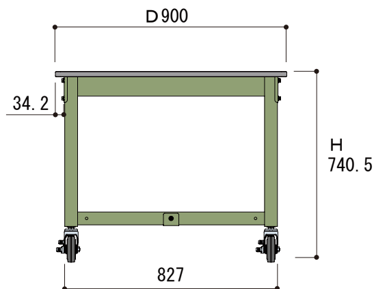
側面図
