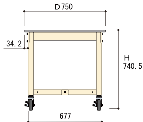
側面図
