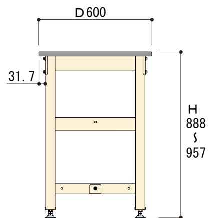
側面図
