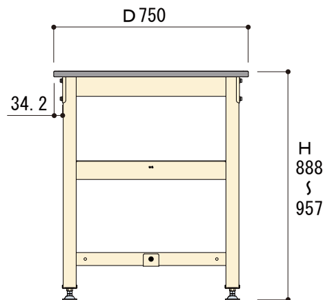
側面図
