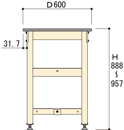
側面図
