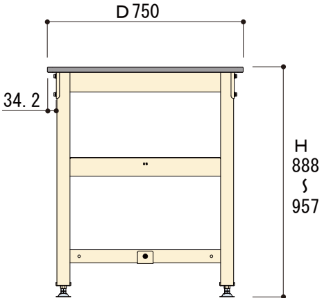
側面図
