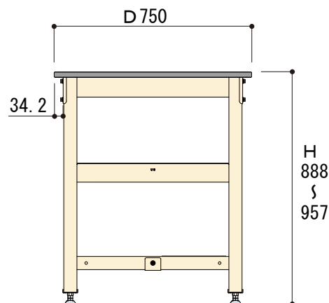
側面図
