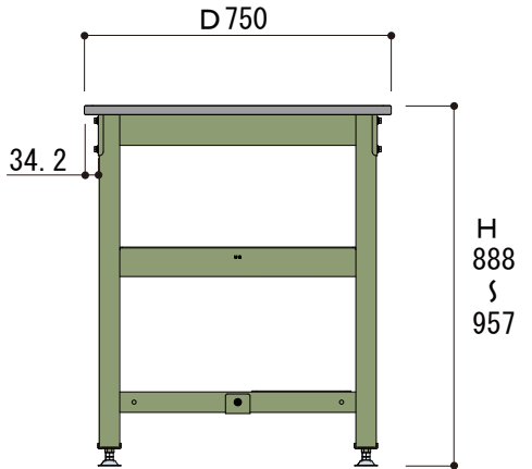
側面図
