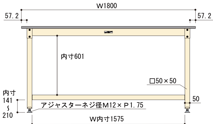
正面図
