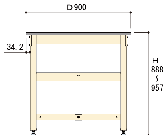
側面図
