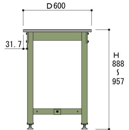
側面図
