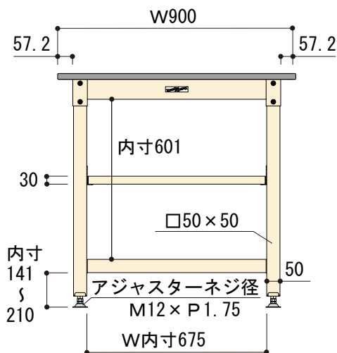
正面図
