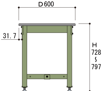
側面図
