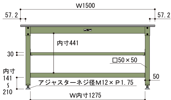
正面図
