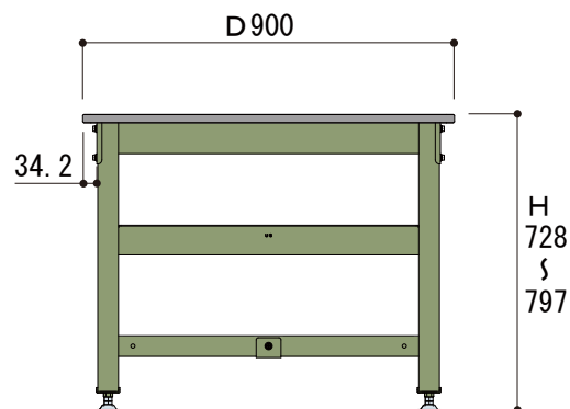
側面図
