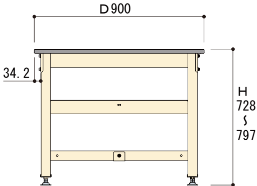
側面図
