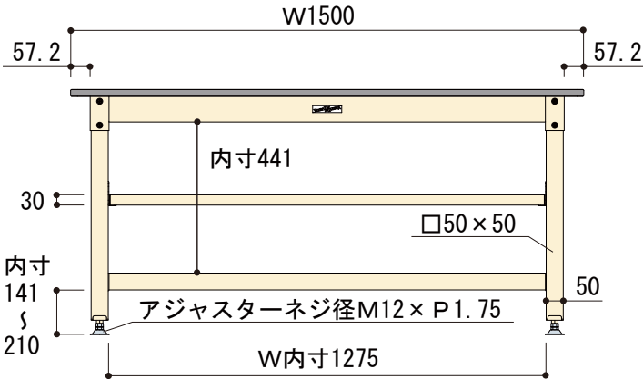
正面図
