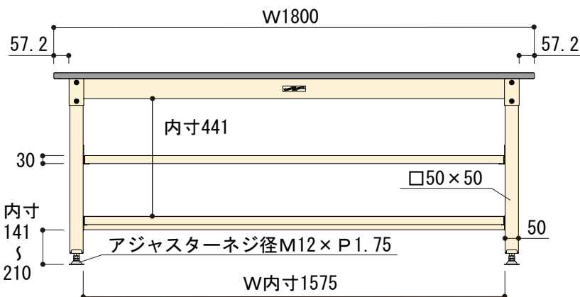
正面図
