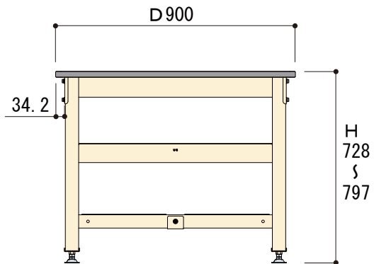
側面図
