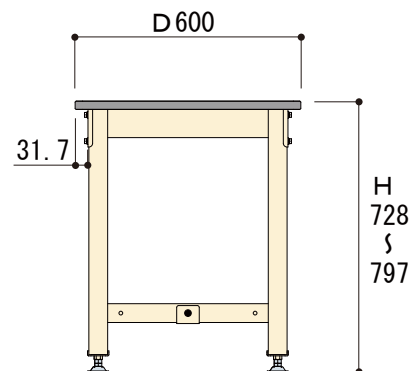
側面図
