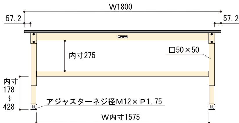
正面図
