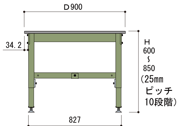
側面図
