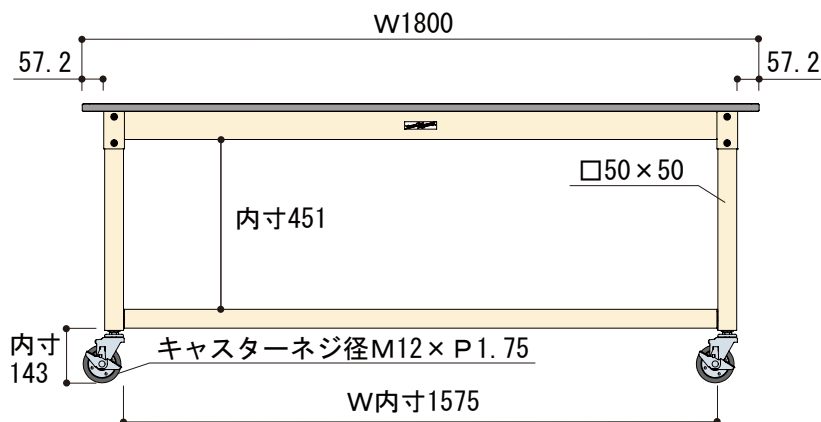
正面図
