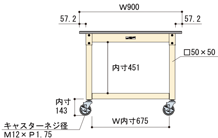
正面図
