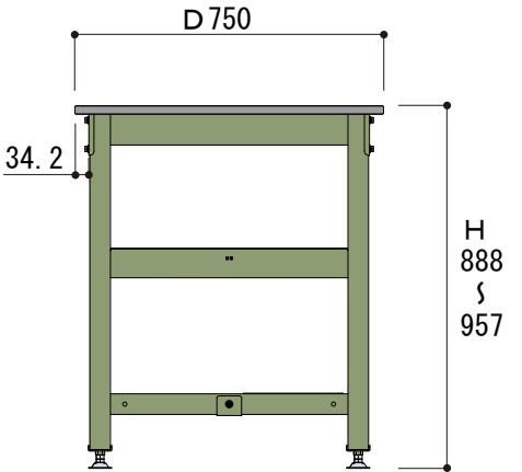
側面図
