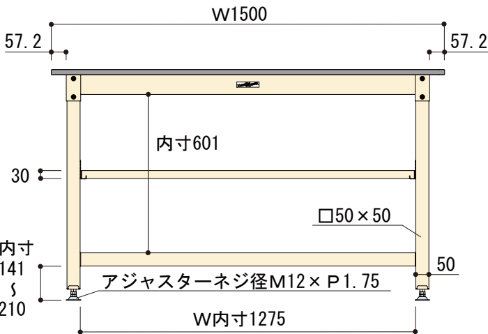
正面図
