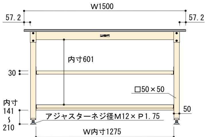
正面図
