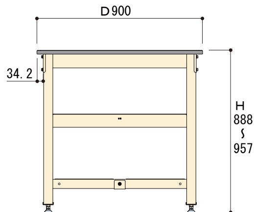
側面図
