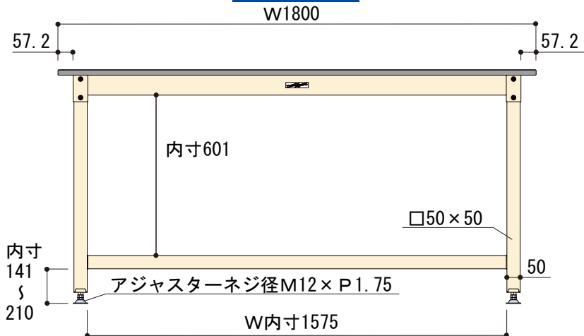
正面図
