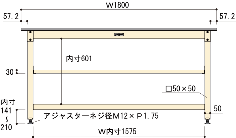
正面図
