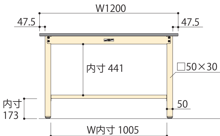
正面図
