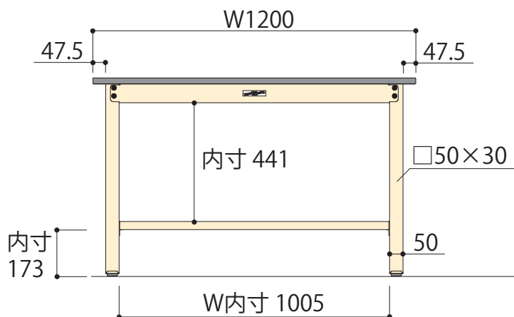
正面図
