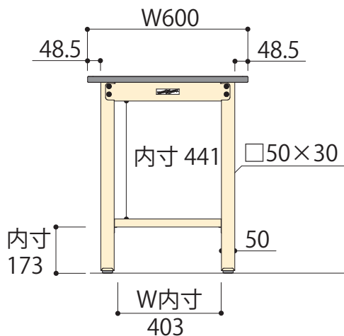
正面図
