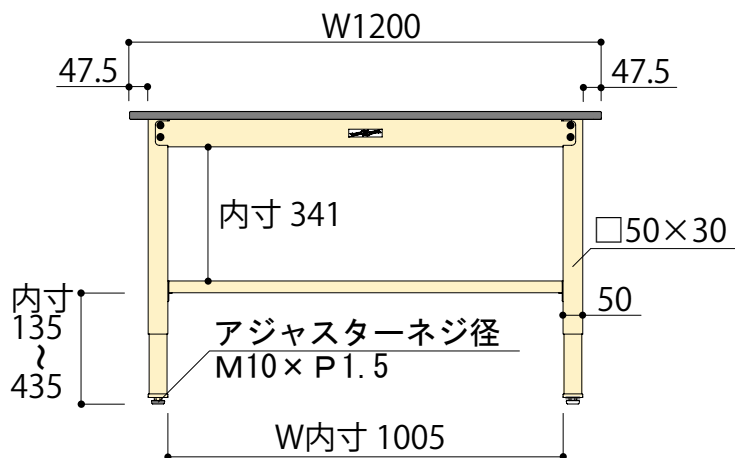
正面図
