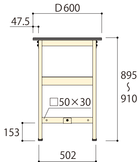
側面図
