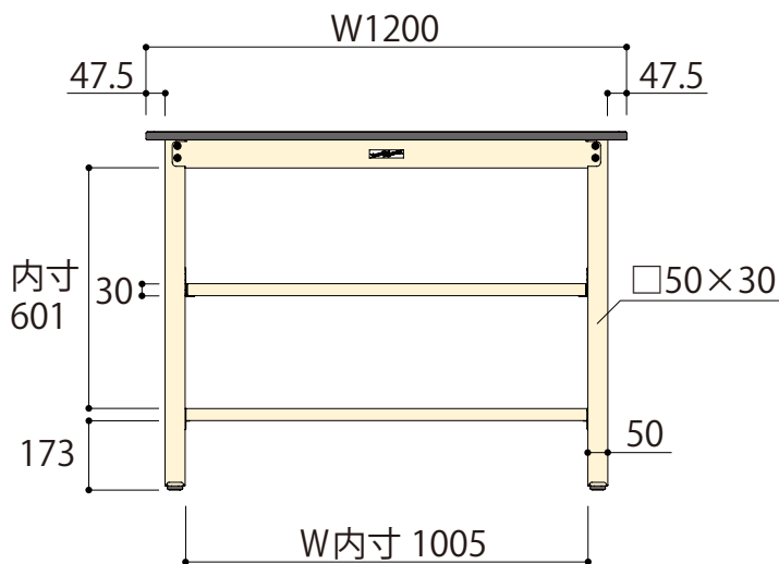
正面図
